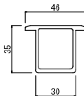
中間固定金具断面
